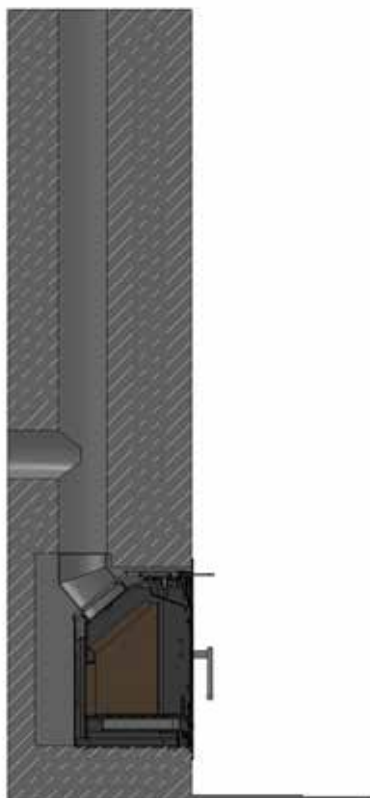
S81-90 tilsluttet eksisterende oppmuret skorstein
