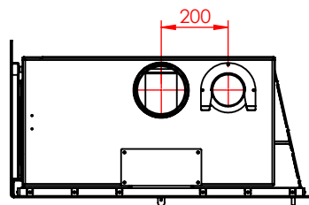
JUPITER 500-850 MED FAST GLAS 1 SIDE, AIRBOX TOP
