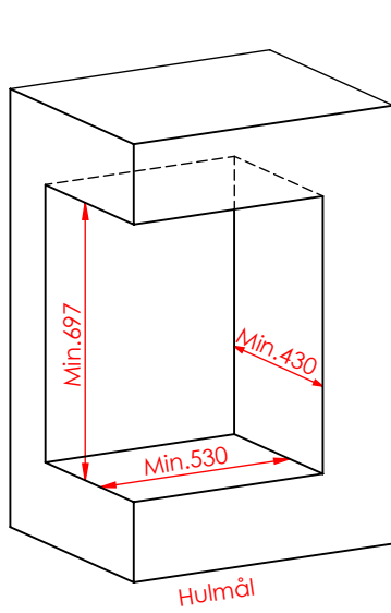
JUPITER 550 HØJFORMAT MED FAST GLAS 1 SIDE
